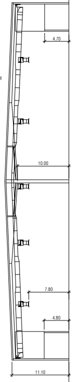
SYSTEMSCHNITT / VERTICAL CROSS SECTION
